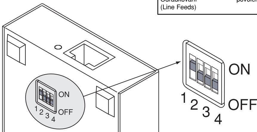
Obrázek 4.14 DIP přepínač č. 1 v pozici „ON“
