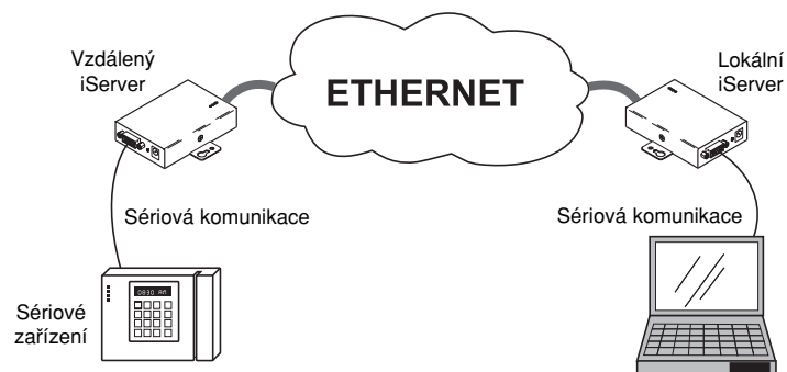
Obrázek 4.22 Komunikace PC se vzdáleným zařízením
