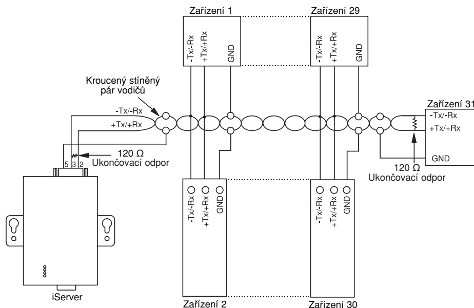
Obrázek 2.5 Zapojení poloduplexní linky RS-485 pro více zařízení
