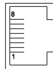
Obrázek 2.6 Konektor RJ45
