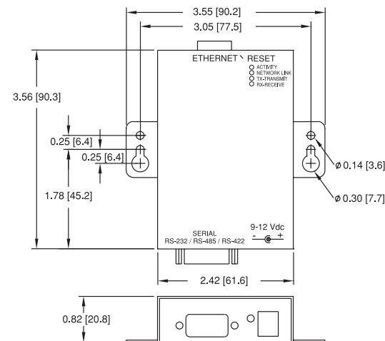
Obrázek 2.1 Montáž
