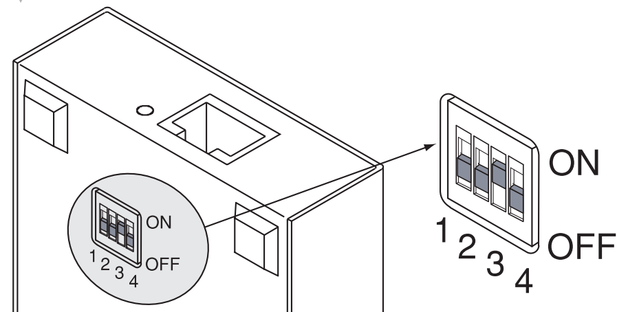
Obrázek 3.2 DIP přepínače na zadní straně krytu iServeru
