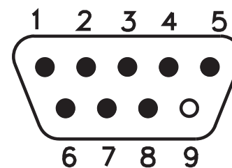
Obrázek 2.4 Konektor DB9
