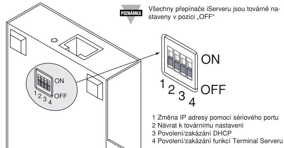
Obrázek 2.2 DIP přepínače
